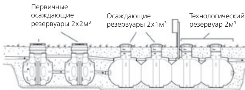
«Urolog»-15 ре для обработки сточных вод дома на три семьи Urolog код 330115
